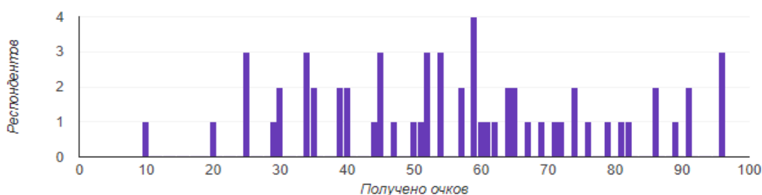
Распределение баллов
